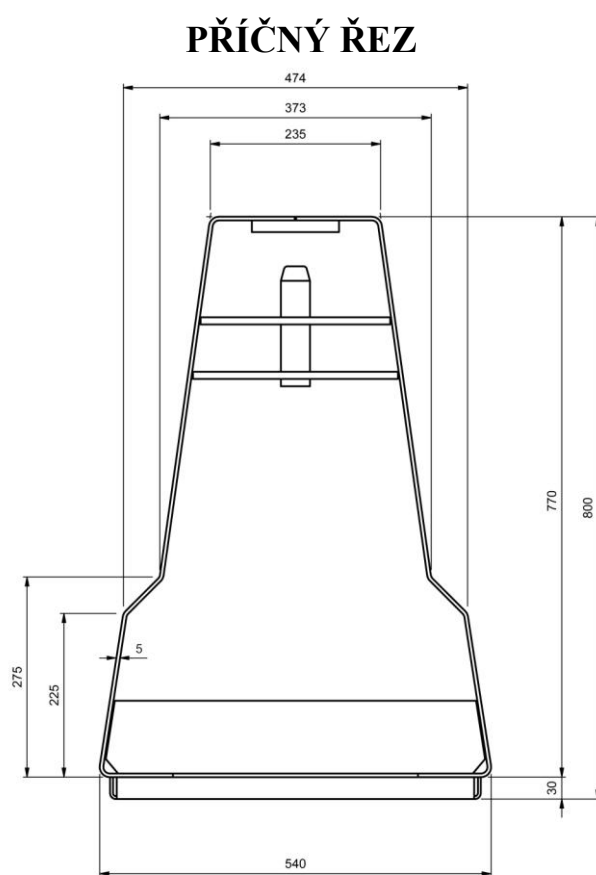
Obrázek 3 – svodidlo BG800
