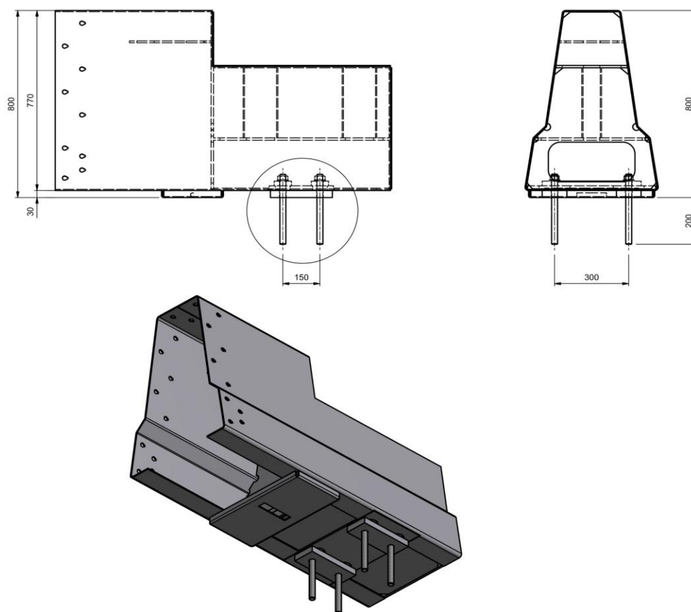
Obrázek 20 – otevírací svodidlo BG800 Opening Gate – detail kotvení pevného dílu
