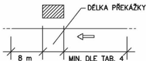
Obrázek 22 – svodidlo BG800 před překážkou a místem nebezpečí
